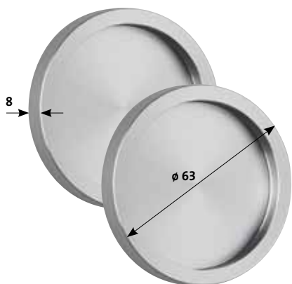
Griffmuschel-Paar Rund Edelstahl gebürstet 41165
