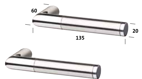
Drückerpaar Quaranta Nickel matt / Chrom 99061
