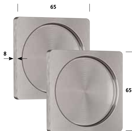
Griffmuschel-Paar Quadratisch Aluminium Edelstahl-Optik 41994
