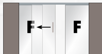
1 Tür mittig, nach links oder rechts öffnend, 2 Elemente links und rechts (F), Breite bis 3390 mm möglich
