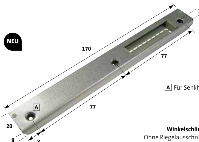
Winkelschließblech abgerundet Ohne Riegelausschnitt, Silber lackiert, DIN Links 99427
