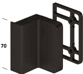
Gegenkasten zu Schiebetürschloss Matt Schwarz Für einflügelige Türanlage Wandmontage, ohne Schrauben Inklusive 1 x Wandabstandsplatte 5 mm 99421
