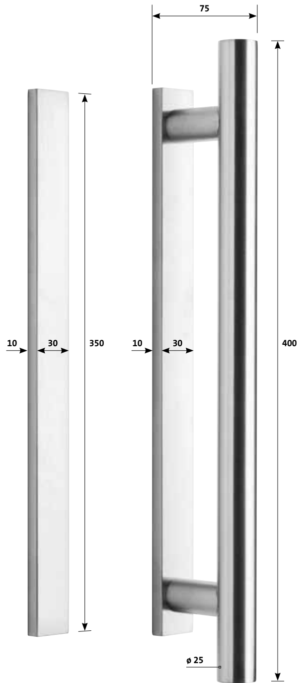
Griffleiste / Griffstange Gerundet Edelstahl gebürstet 41111
