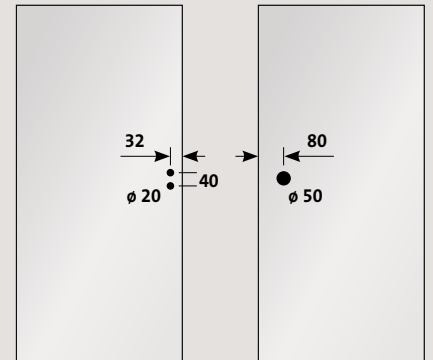
Gegenkasten zu Schiebetürschloss
