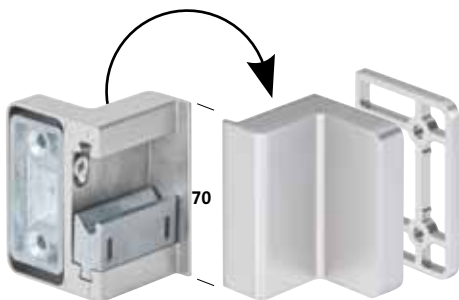
Gegenkasten zu Schiebetürschloss Edelstahl gebürstet Für einflügelige Türanlage Wandmontage, ohne Schrauben Inklusive 1 x Wandabstandsplatte 5 mm 99415
