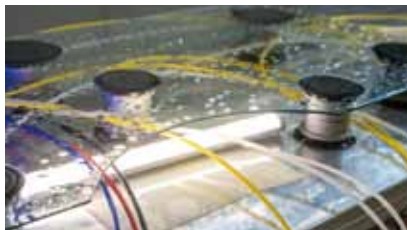
CNC-Glasausschnitte und Bohrungen
