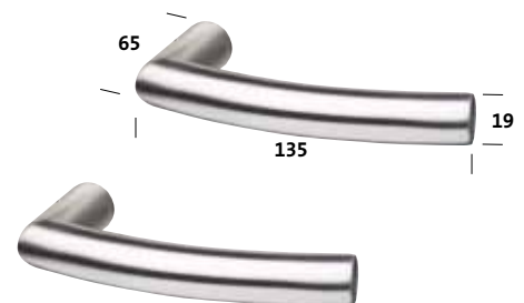
Drückerpaar Due Edelstahl gebürstet 99017
