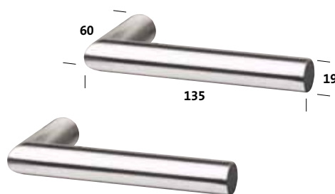
Drückerpaar Uno Edelstahl gebürstet 99016
