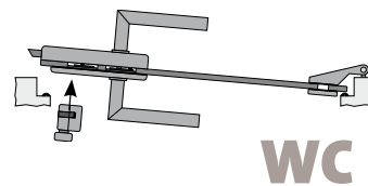
WC-Zylinder für nach außen öffnende Tür Einsetzbar in Schlosskasten PZ, WC-Zylinder an Schlossgegensseite 99035
