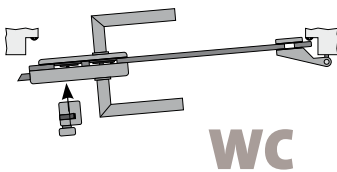
WC-Zylinder für nach innen öffnende Tür Einsetzbar in Schlosskasten PZ, WC-Zylinder an Schlossseite 99034
