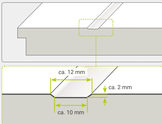
Lines straight | Querschnitt
