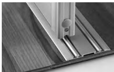
Die Bodenrollen sind „unsichtbar“ im Sockelprofil verbaut
