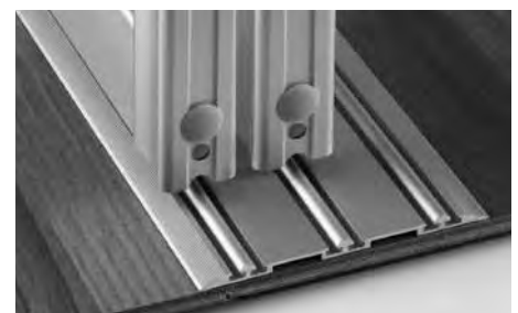
Leichtgängig gleiten die Türen über die Bodenschiene
